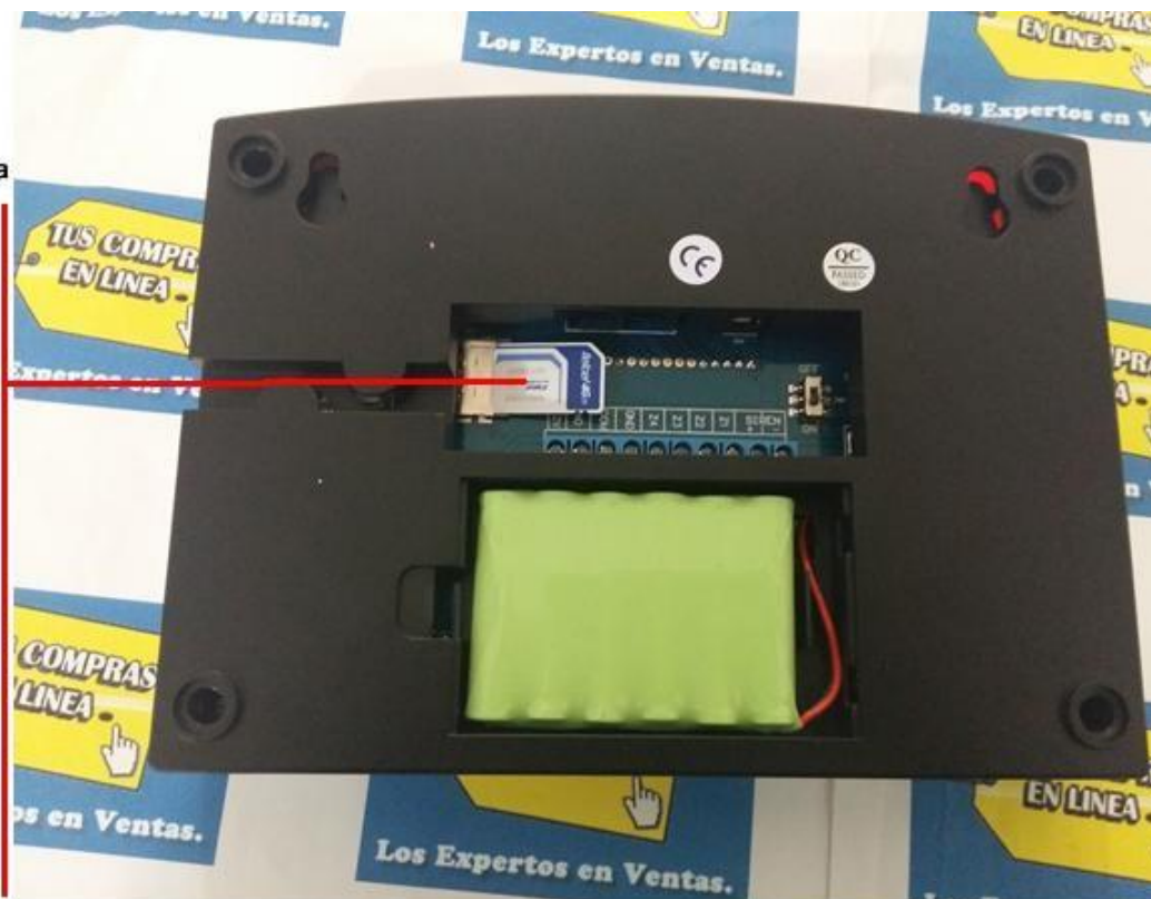
Nano SIM
